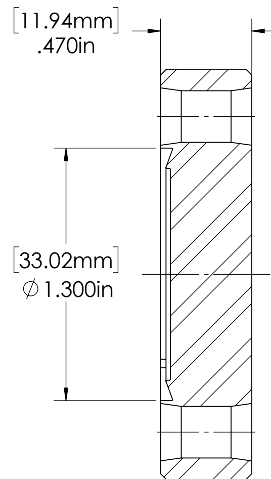
SECTION A-A
