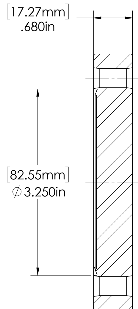
SECTION A-A
