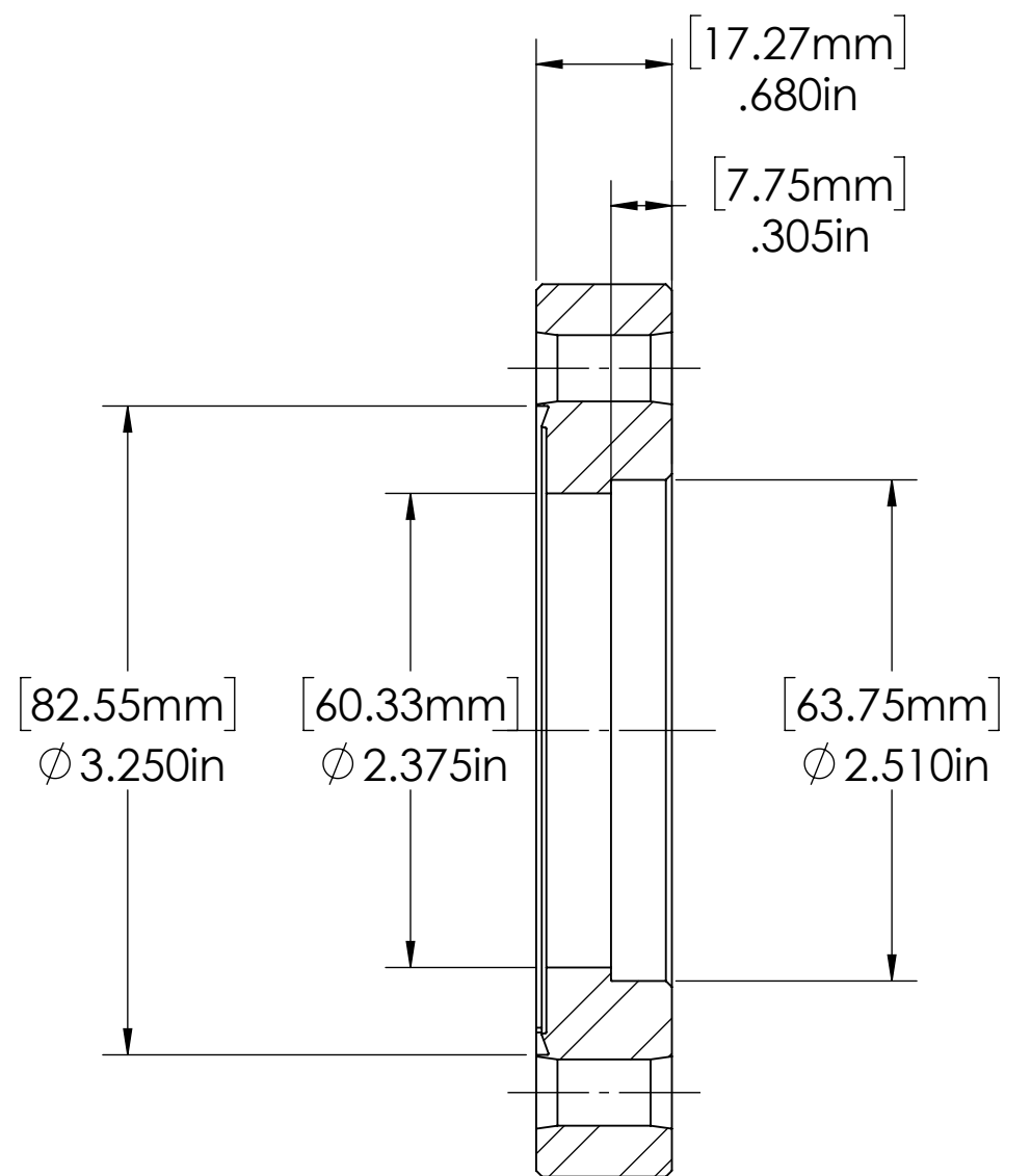
SECTION A-A
