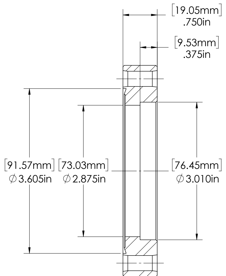
SECTION A-A
