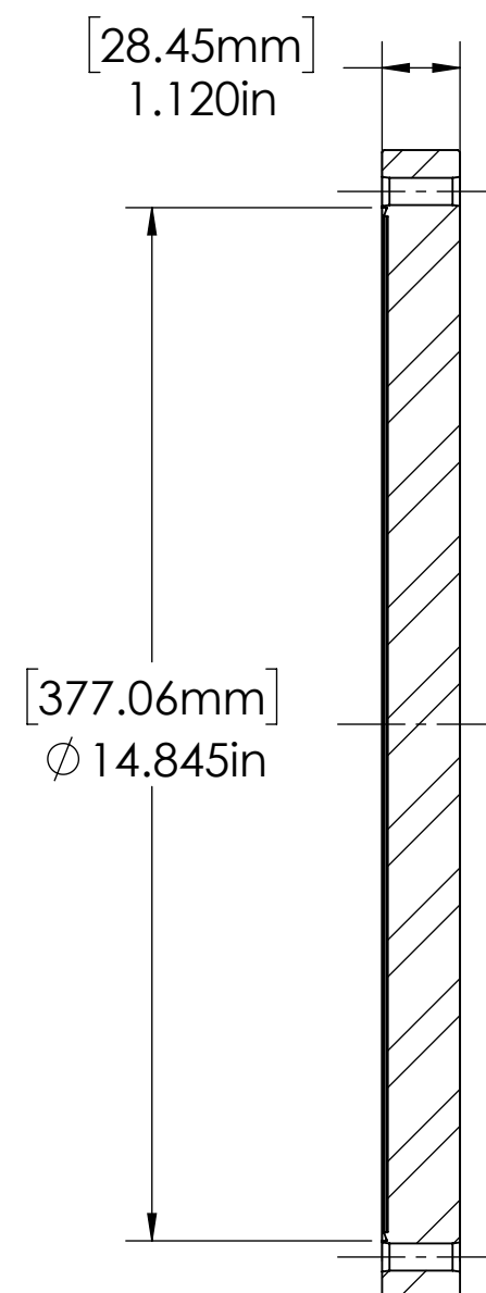
SECTION A-A
