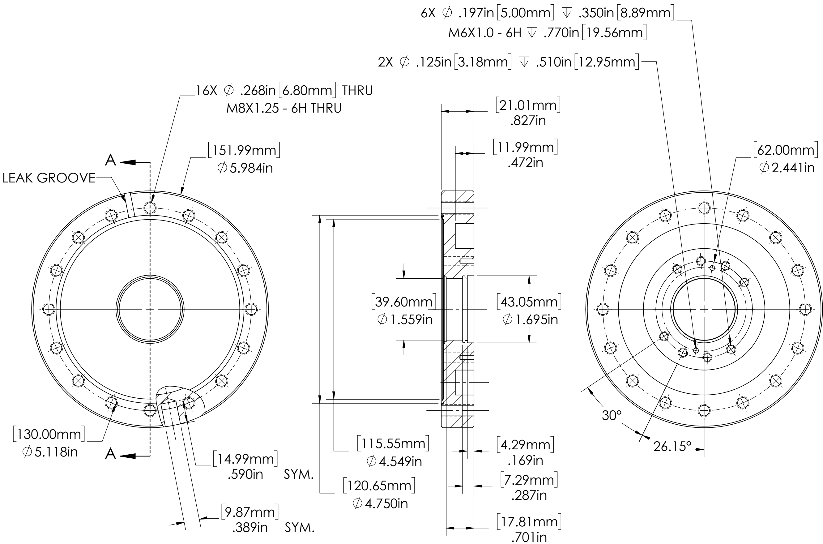
SECTION A-A
