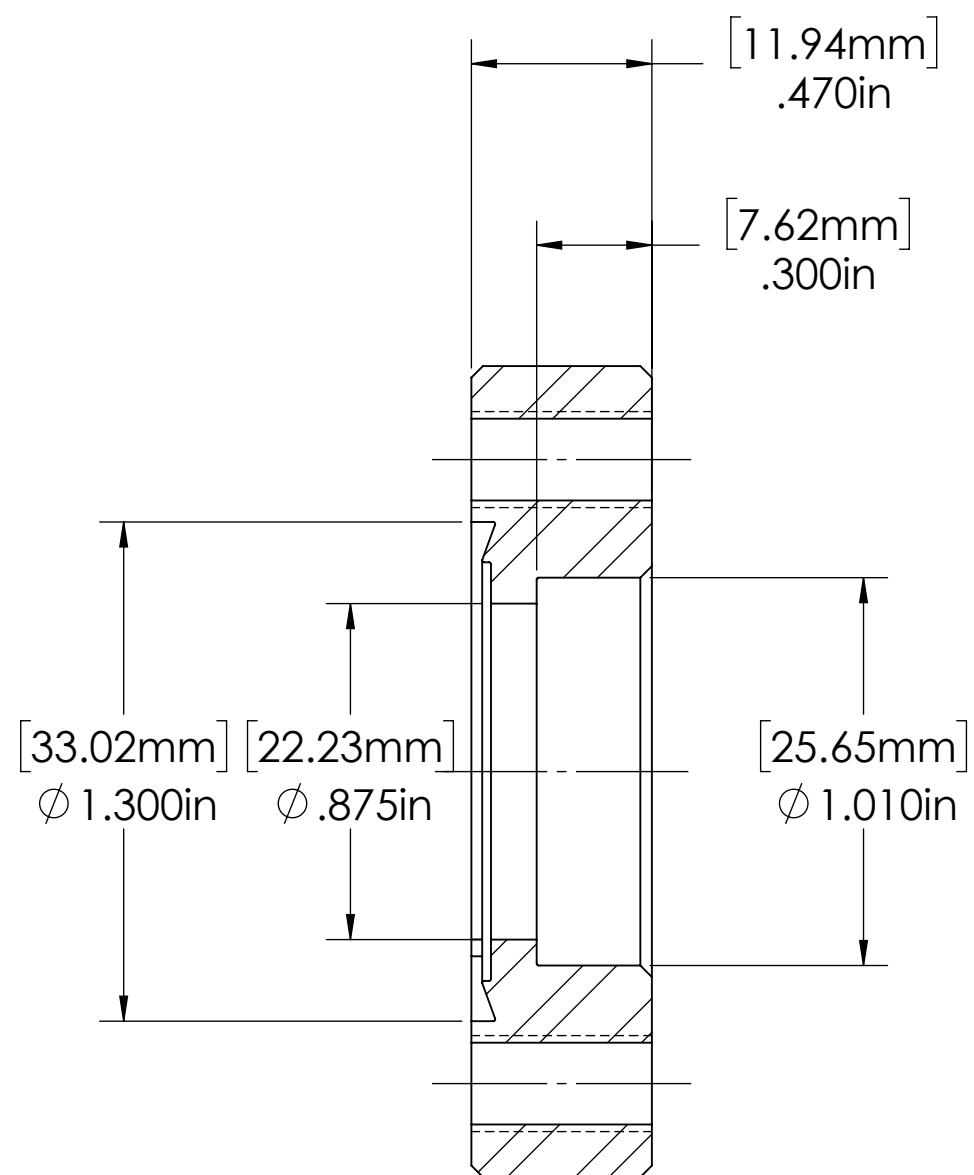
SECTION A-A
