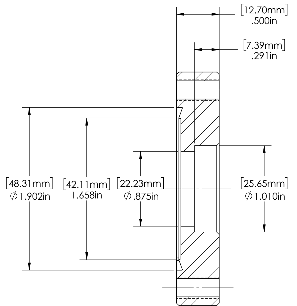
SECTION A-A
