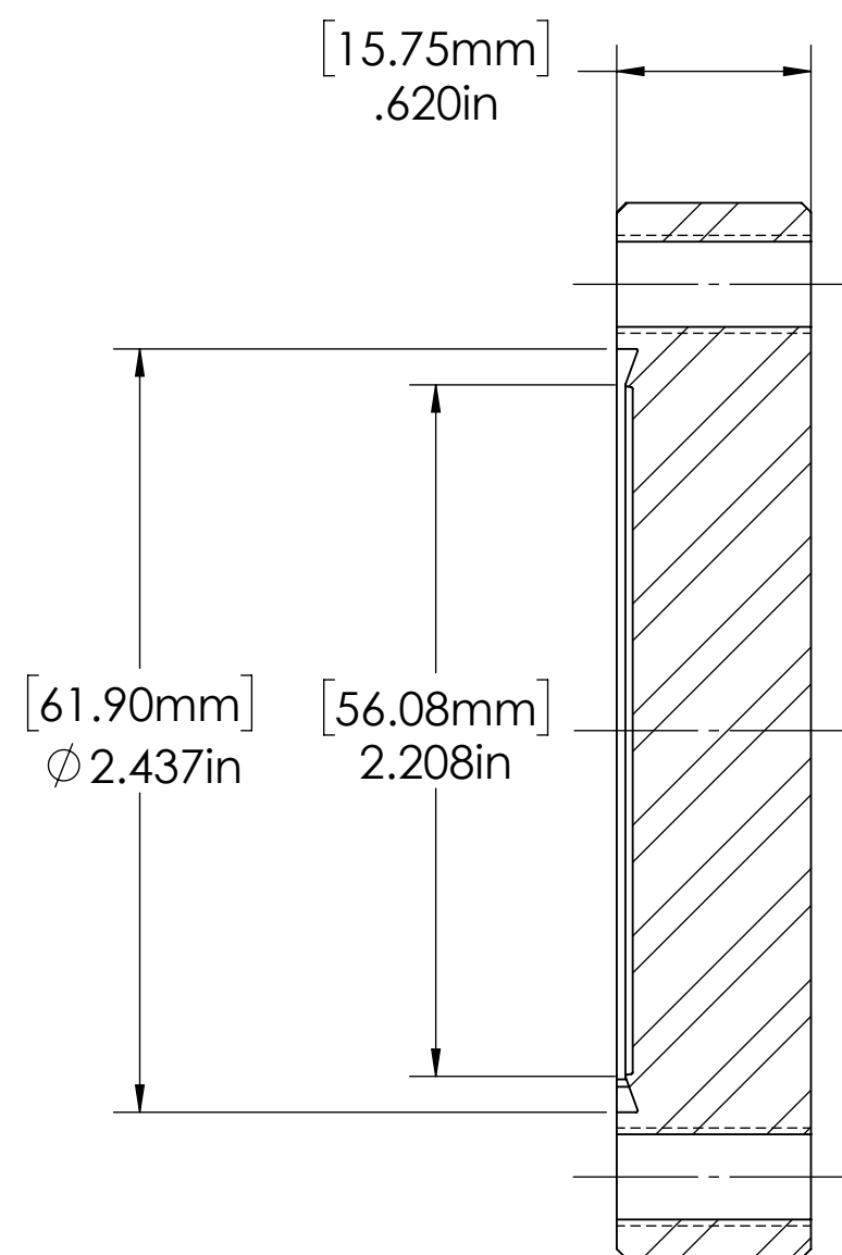
SECTION A-A
