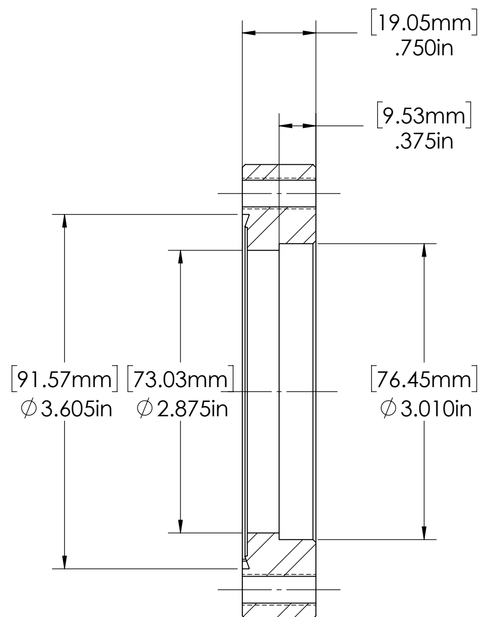
SECTION A-A
