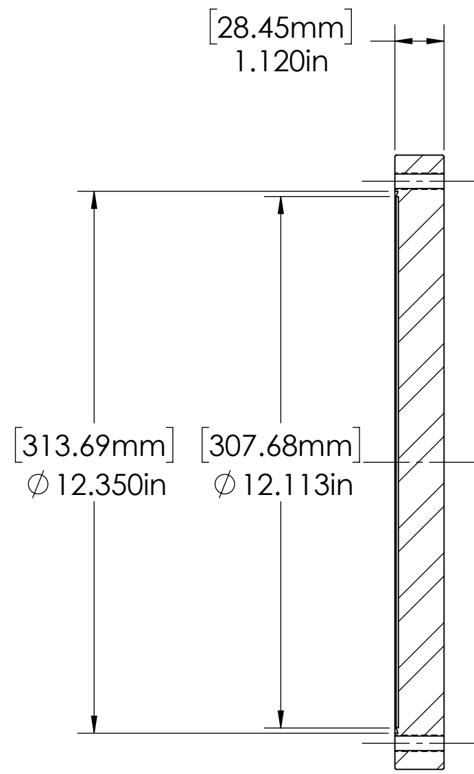
SECTION A-A
