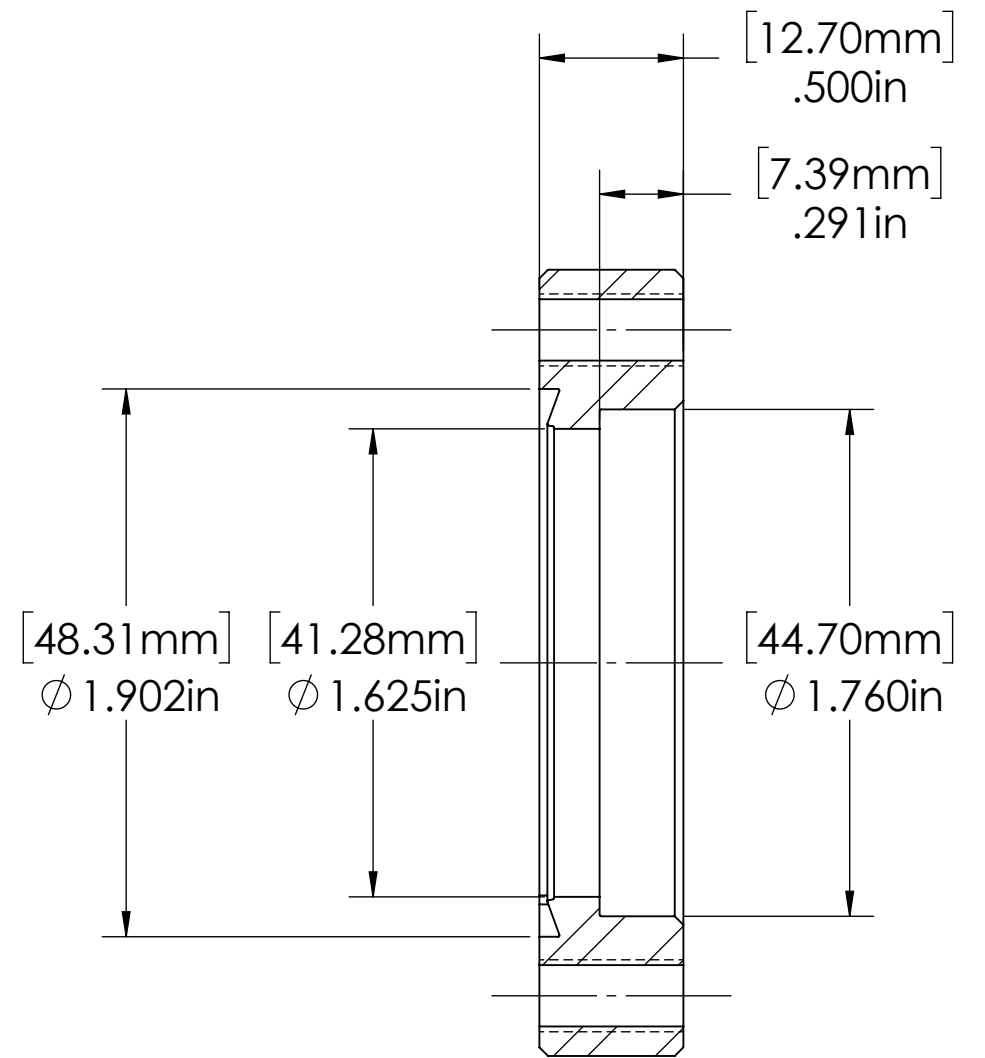
SECTION A-A
