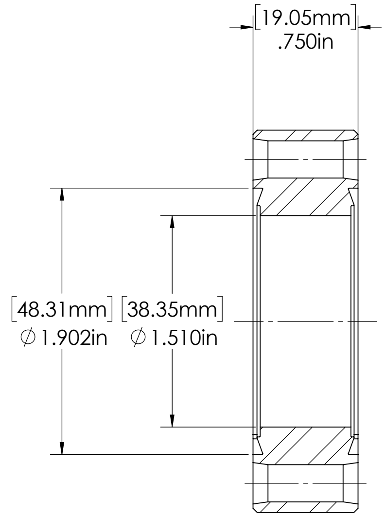
SECTION A-A
