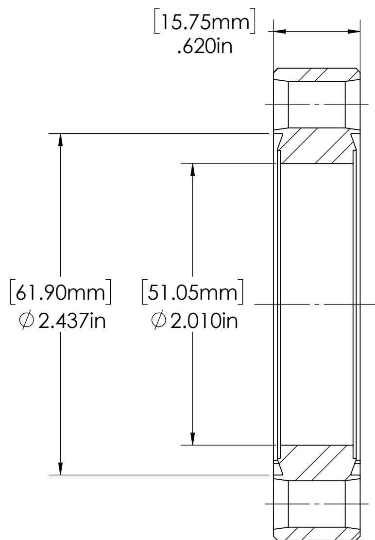
SECTION A-A
