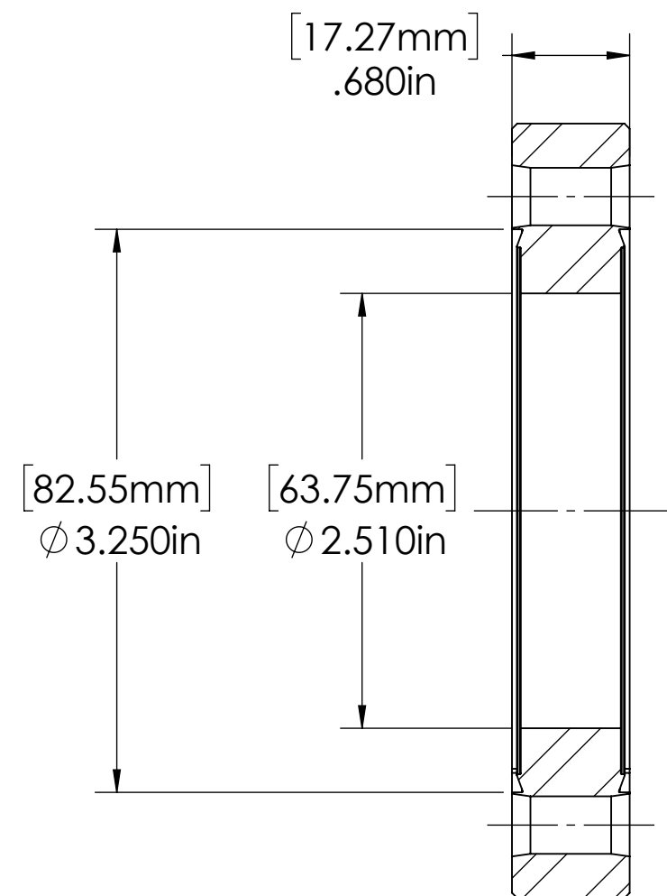
SECTION A-A
