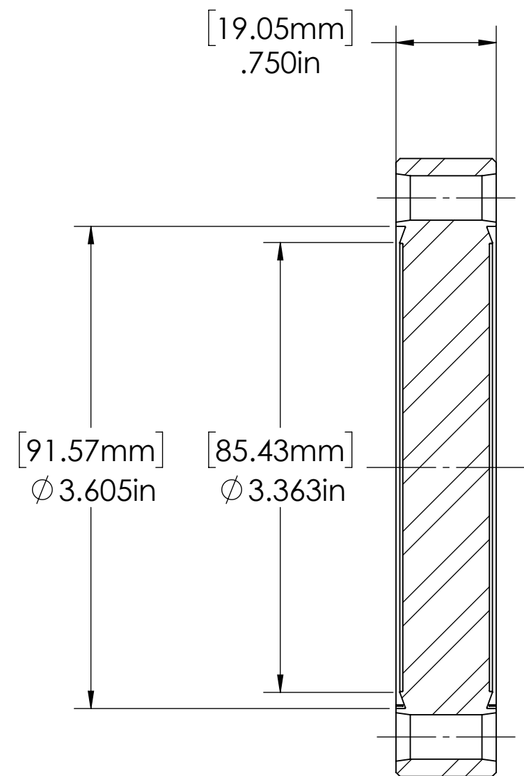
SECTION A-A
