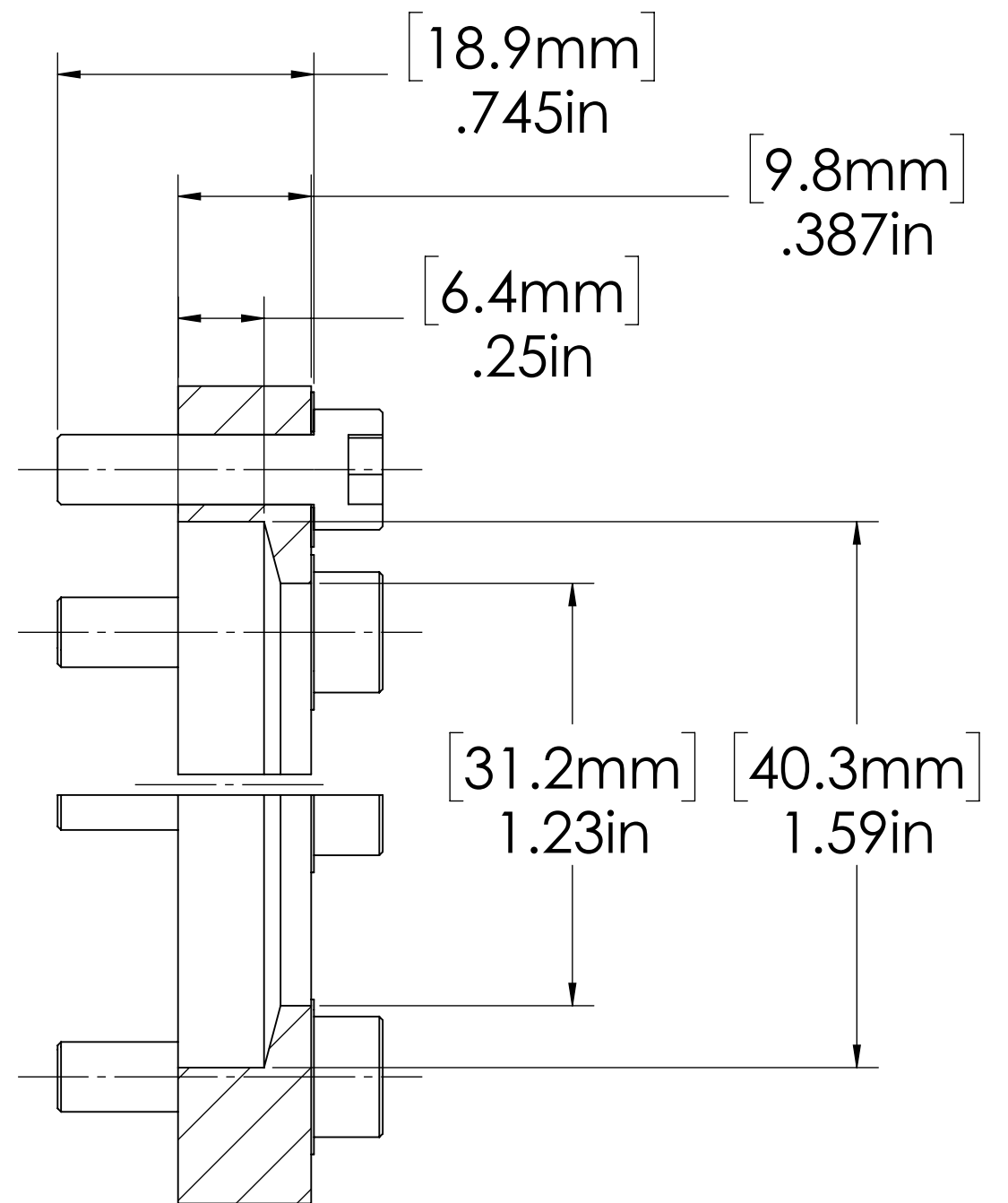
SECTION A-A
