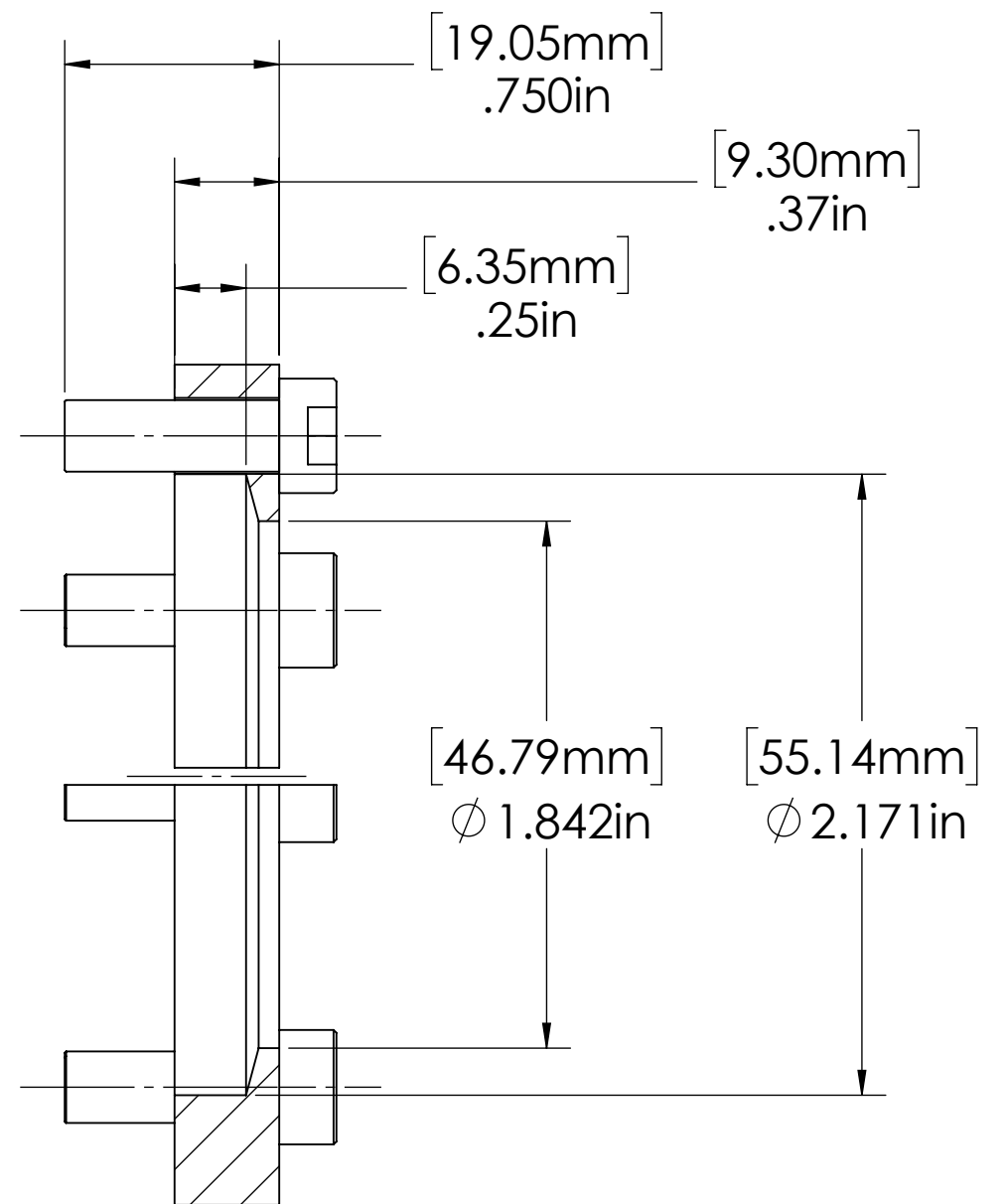
SECTION A-A
