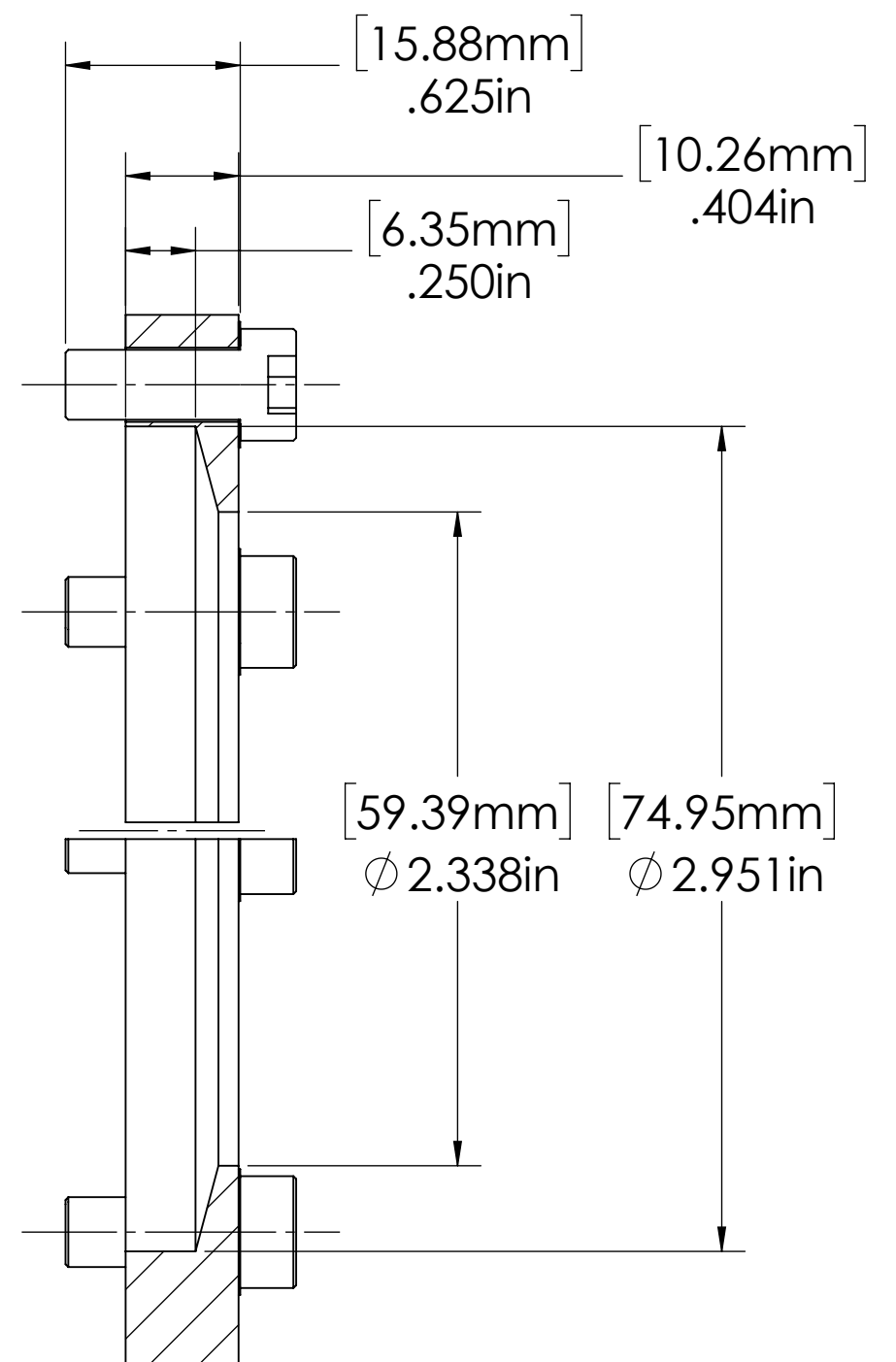
SECTION A-A
